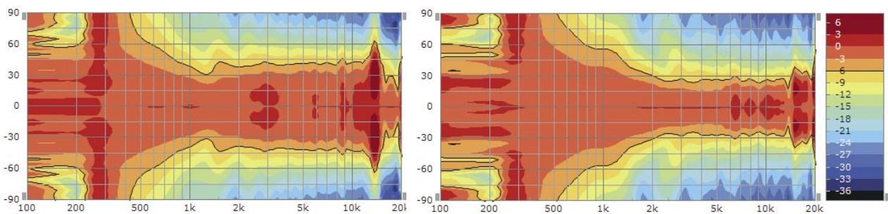
horizontale und vertikale Isobaren 1/10 oct. smoothing
