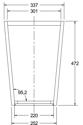
Schnitt TT
